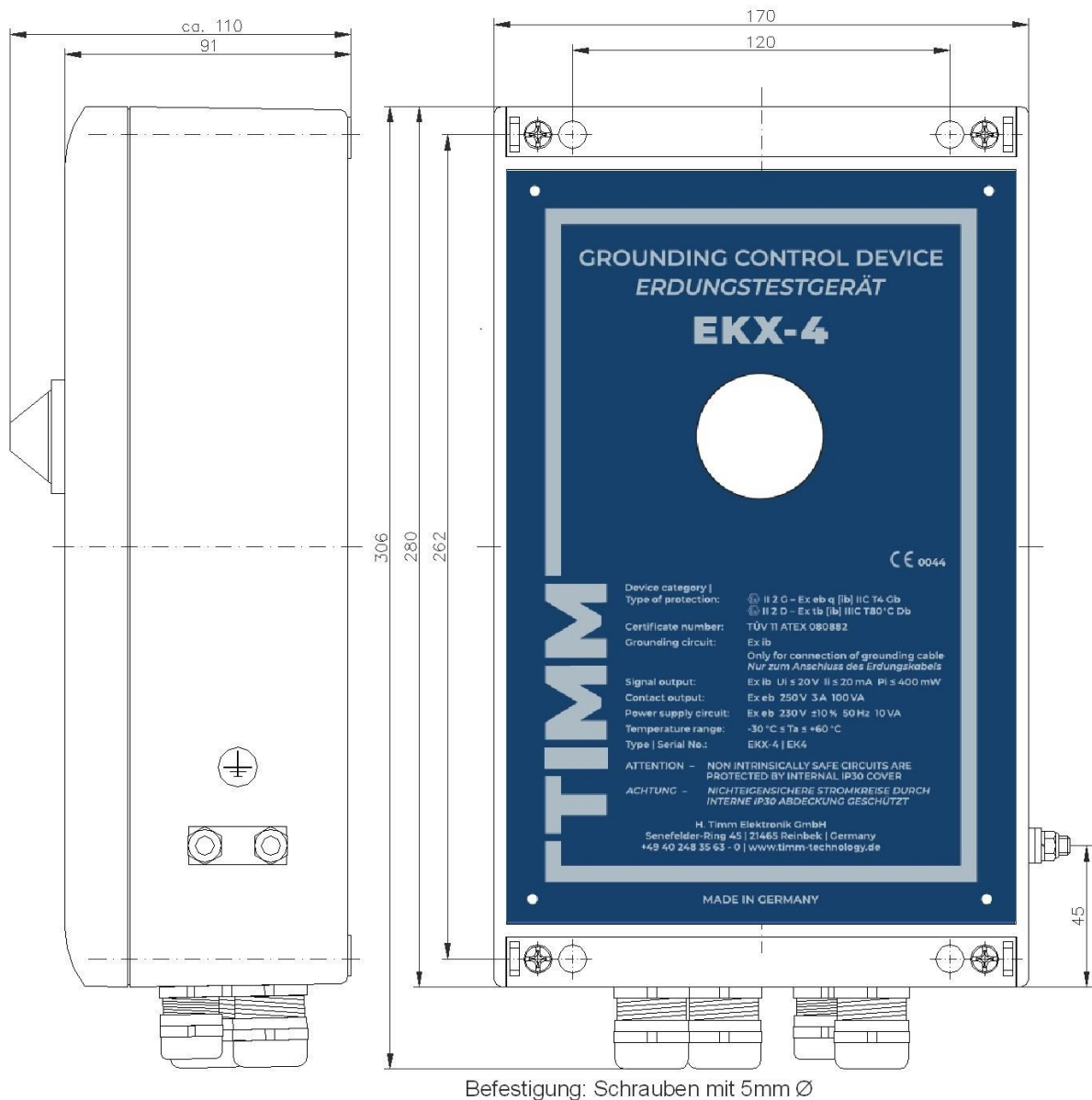
1. Maßbild
