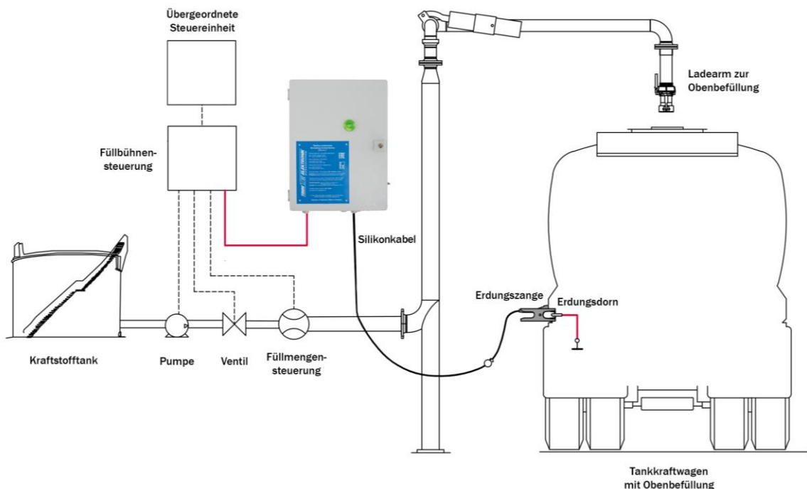
Überwachte Erdung eines Straßentankfahrzeugs mit dem Erdungstestgerät EKX-4 LT
