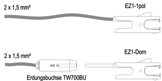
Ausführungen der Erdungszange EZ1
