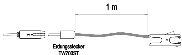
Steckverbindung aus Buchse TW700BU und Stecker TW700ST mit 1 m Kabel zur Erdungszange
