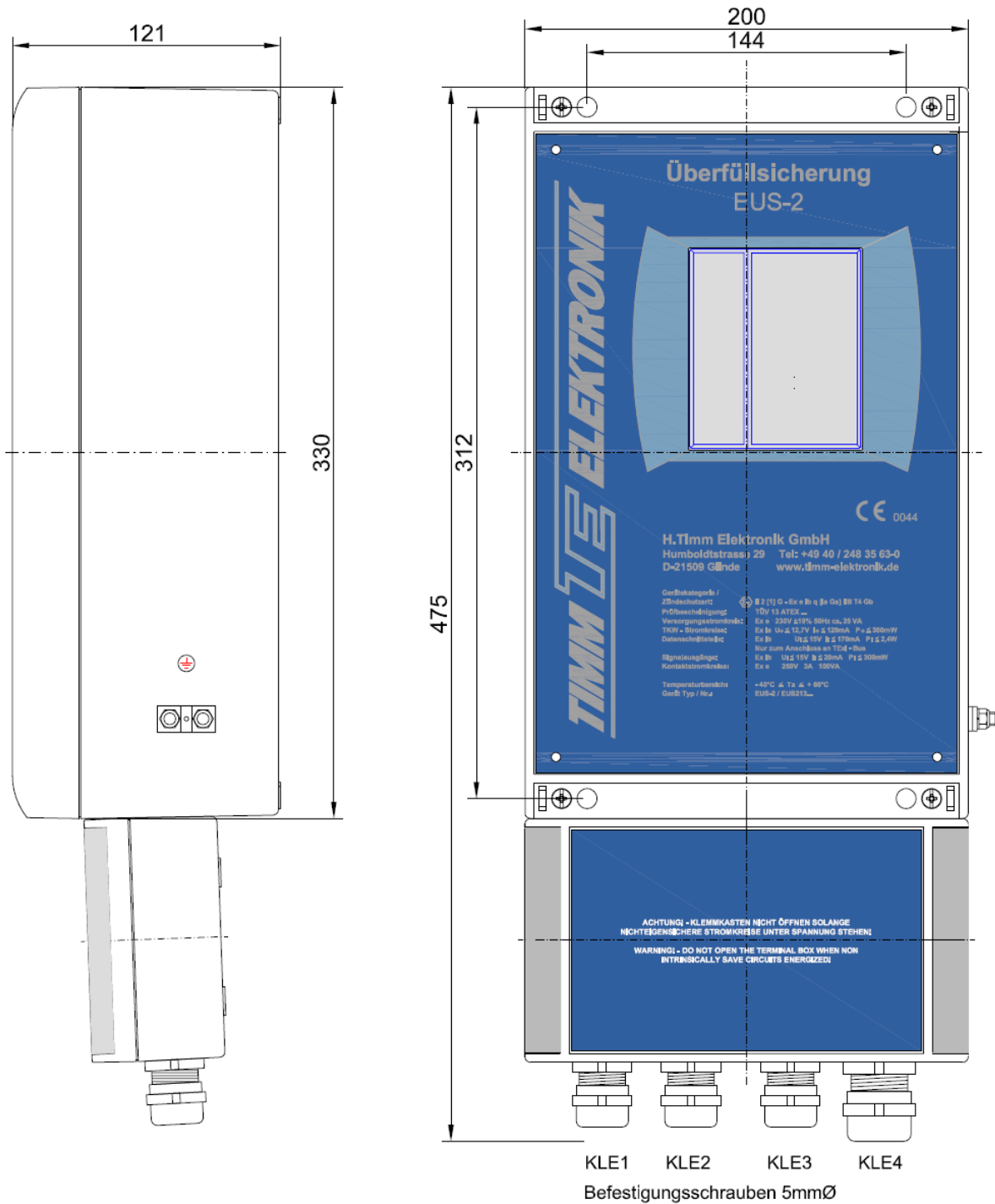
1. Maßbild
